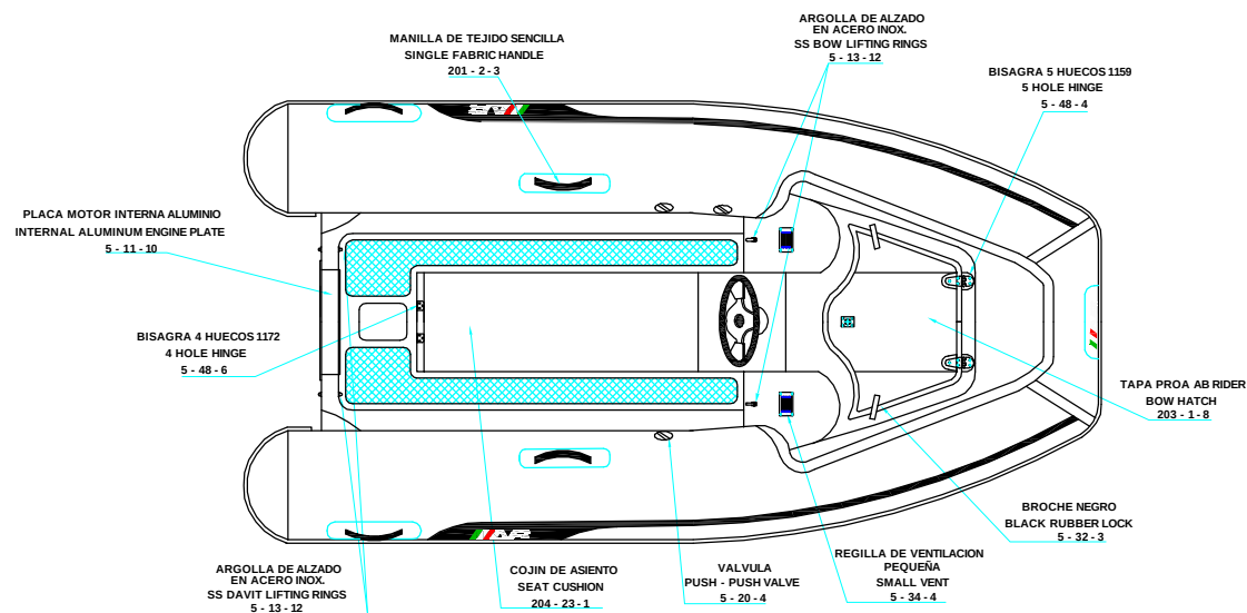
PLANT VIEW VISTA EN PLANTA
